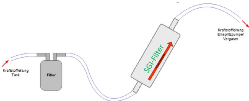
Bild 1. Schematische Darstellung Einbau des SGI-Filters
